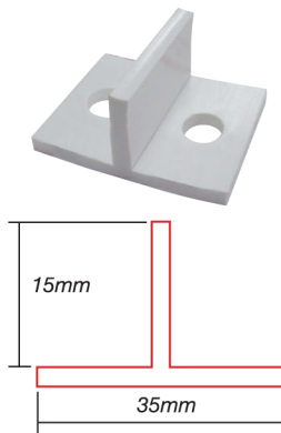
TT1 TRANSITION T-PROFILE 15X35MM
